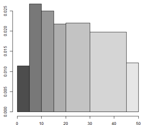
Figura 1.4: Histograma.
