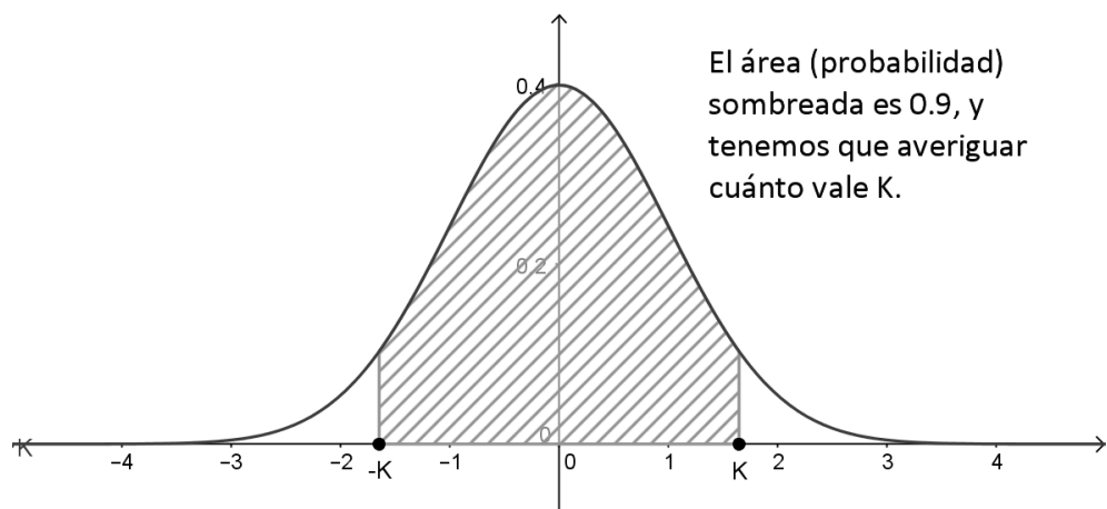
Figura 6.7: El paso clave en la construcción de un intervalo de confianza al 90 %.
