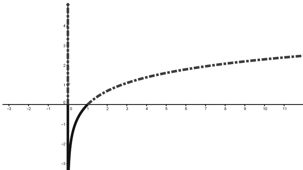
Figura 9.9: El logaritmo, y su efecto como transformación de datos.
