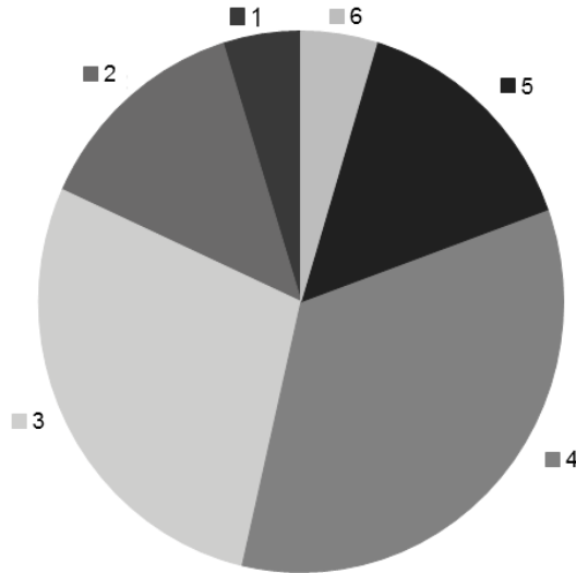
Figura 1.2: Diagrama de sectores circulares, dibujado con Calc.
