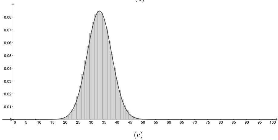
Figura 5.3: (a) La distribución de probabilidad binomial B(10, \frac{1}{3}) . (b) La distribución de probabilidad binomial B(100, \frac{1}{3}) . (c) La misma distribución B(100, \frac{1}{3}) , con una curva “misteriosa” superpuesta.
