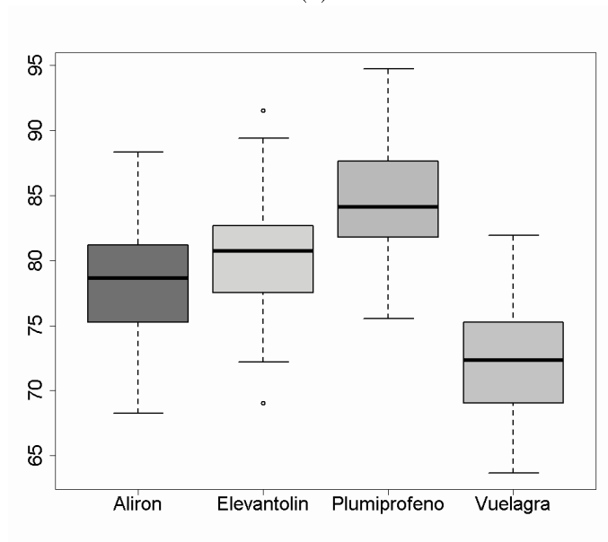
Figura 11.2: (a) Histogramas y (b) diagramas de cajas paralelos para la condición de normalidad.
