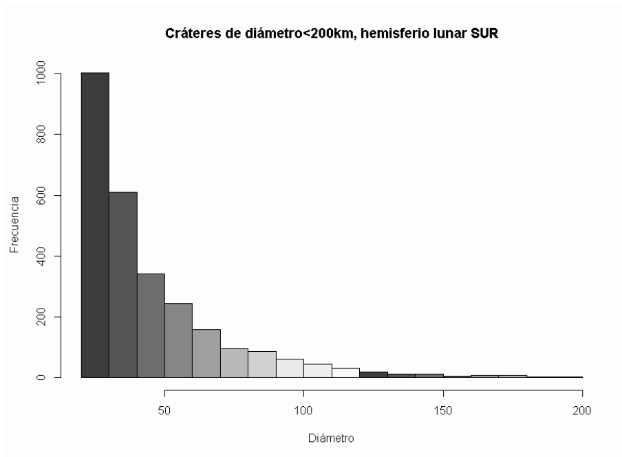
Figura 9.1: Distribución de diámetros (< 200 km), de cráteres del hemisferio sur lunar
