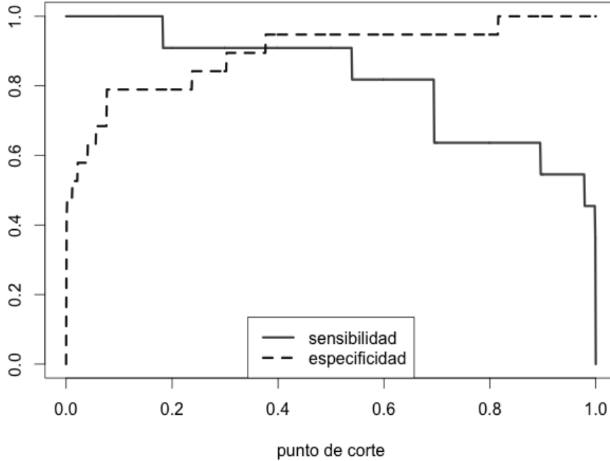
Figura 13.16: Sensibilidad y especificidad en función del punto de corte c_p en el Ejemplo 13.7.8.
