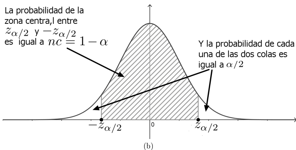
Figura 6.8: Representación gráfica de los valores críticos de la normal estándar Z : (a) significado de z_p para cualquier p , (b) significado del valor z_{\alpha/2} que se usa en los intervalos de confianza para \mu .
