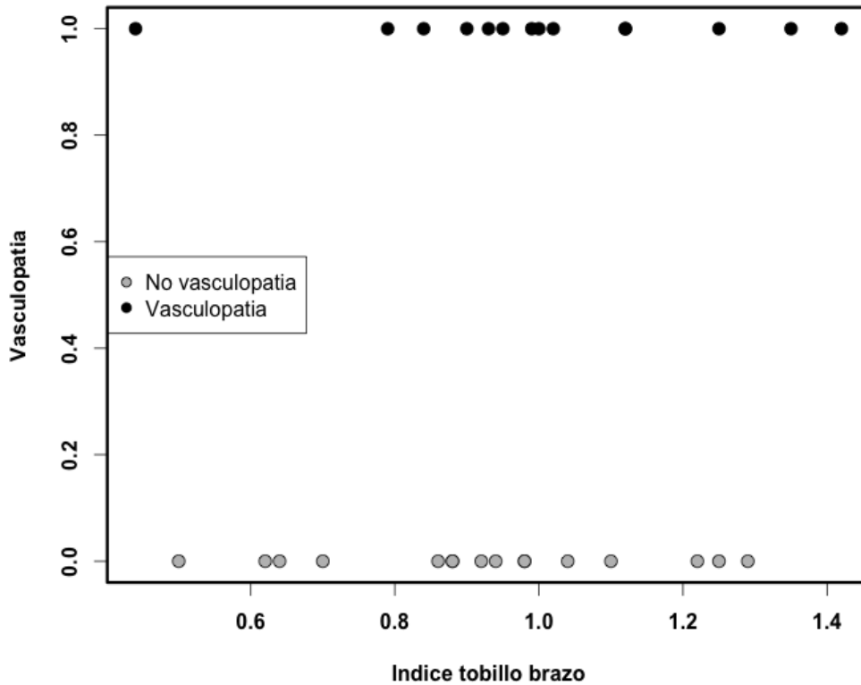
Figura 13.5: El caso “todo ruido, nada de modelo” en el Ejemplo 13.1.4.
