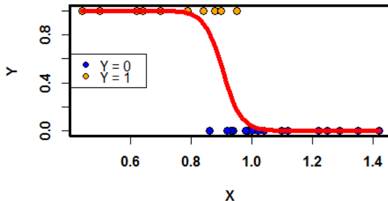
Figura 13.13: Curva logística para los datos itb / vasculopatía, en el Ejemplo 13.3.4.
