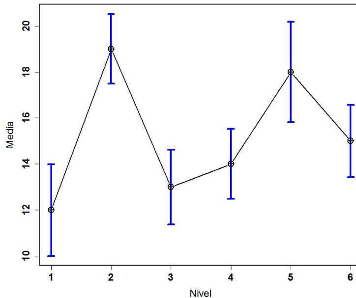
Figura 11.6: Intervalos de confianza (ajustados por Bonferroni) para las medias del Ejemplo 11.6.4.
