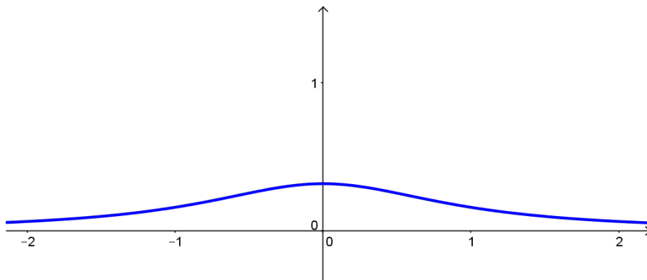
Figura 5.8: Un ejemplo de función de densidad para una variable aleatoria continua.
