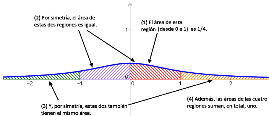
Figura 5.12: Cálculo de probabilidad mediante descomposición en intervalos simétricos.
