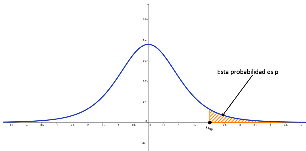
Figura 6.11: El valor crítico t_{k;p} de la distribución T_k de Student.
