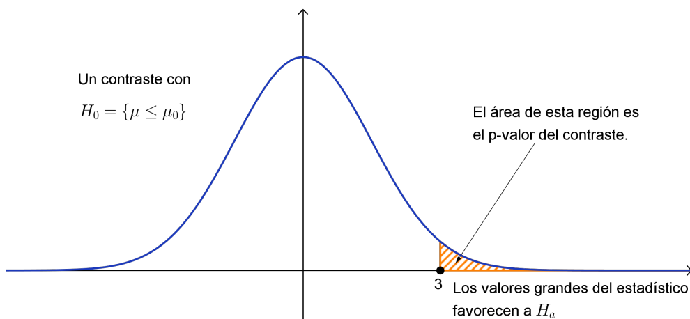
Figura 7.1: Cálculo del p-valor en el Ejemplo 7.2.1.
