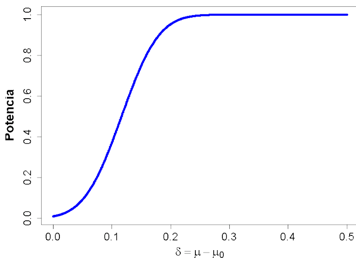
Figura 7.2: Curva de potencia para un contraste de hipótesis con H_0 = \{\mu \leq \mu_0\} , siendo n = 100 , \alpha = 0.01 y s = 0.5 .
