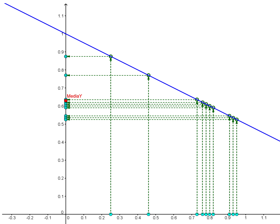
Figura 10.15: Anova en la regresión. Caso “no ruidoso”, en el que la dispersión de los valores y_i se explica completamente por el efecto de la recta.
