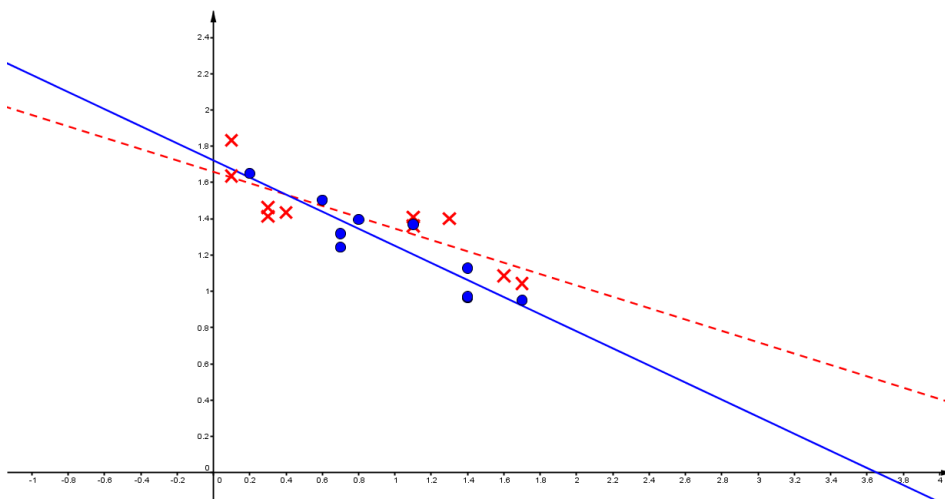
Figura 10.17: Rectas de regresión para dos muestras de una misma población.
