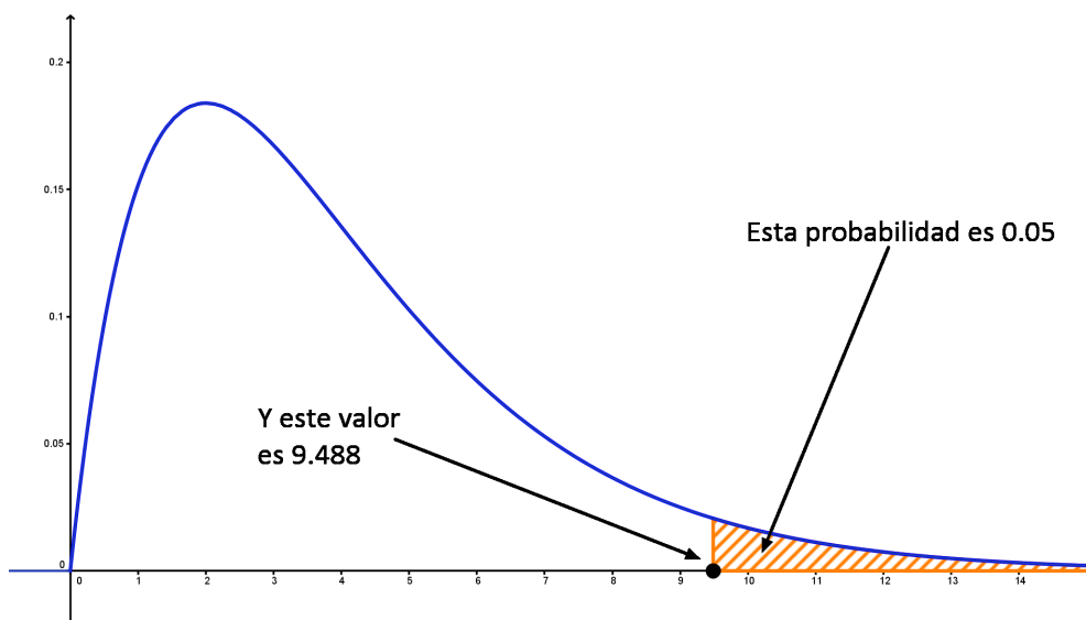
Figura 6.14: Problema inverso de probabilidad ( p_0 = 0.05 ) para \chi^2_4 , cola derecha.
