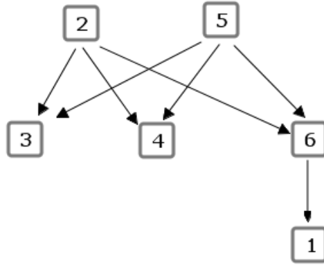
Figura 11.5: Relación de orden parcial entre las medias del Ejemplo 11.6.4.
