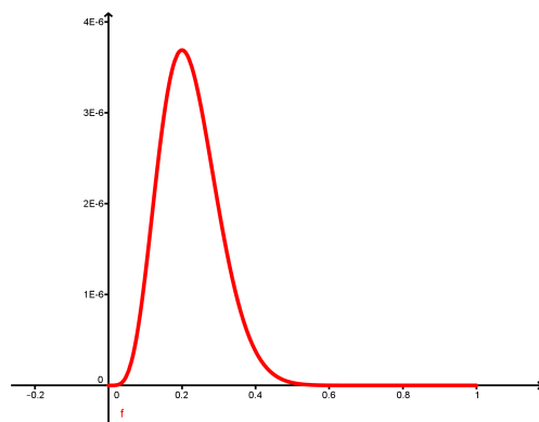
Figura 6.16: Función de verosimilitud \mathcal{L} del Ejemplo 6.7.2.
