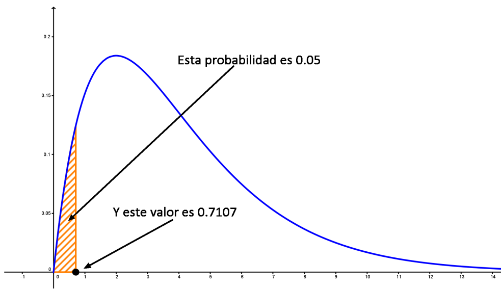
Figura 6.13: Problema inverso de probabilidad ( p_0 = 0.05 ) para \chi_4^2 , cola izquierda.
