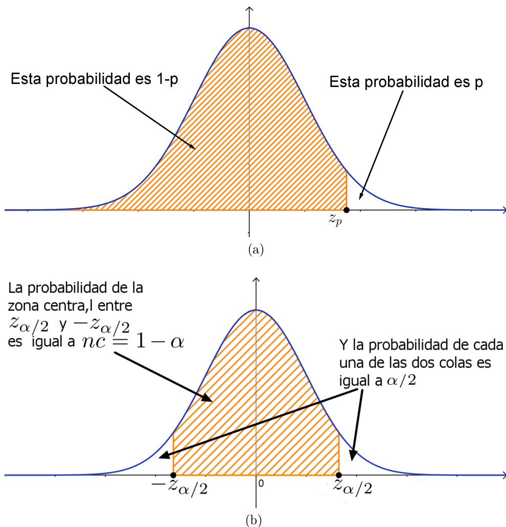
Figura 6.8: Representación gráfica de los valores críticos de la normal estándar Z : (a) significado de z_p para cualquier p , (b) significado del valor z_{\alpha/2} que se usa en los intervalos de confianza para \mu .
