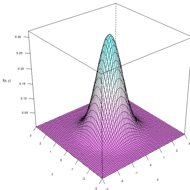
Figura 5.27: Función de densidad del Ejemplo 5.7.1. Atención a las escalas de los ejes, no son todas iguales.
