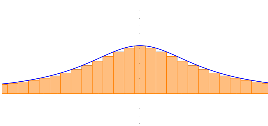
Figura 5.16: Discretizando una variable aleatoria continua
