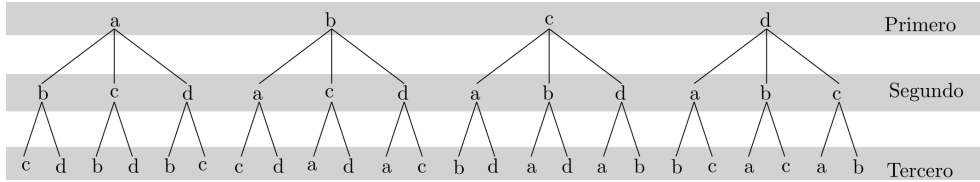
Figura 3.9: Posibles tres primeros puestos.
