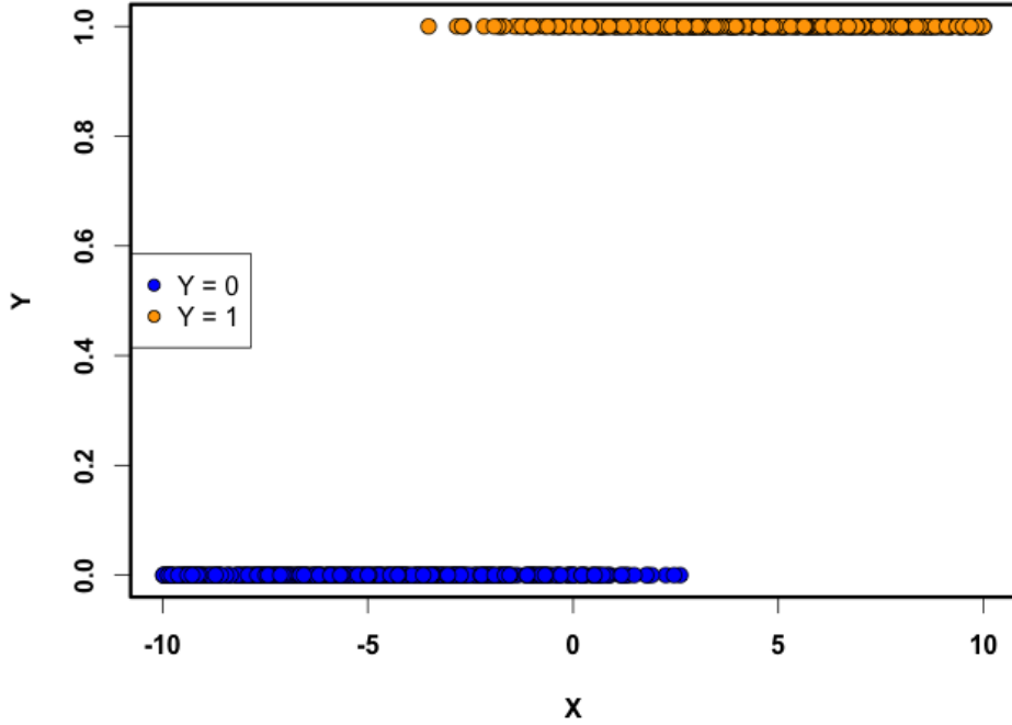
Figura 13.6: Datos muestrales del Ejemplo 13.1.5.
