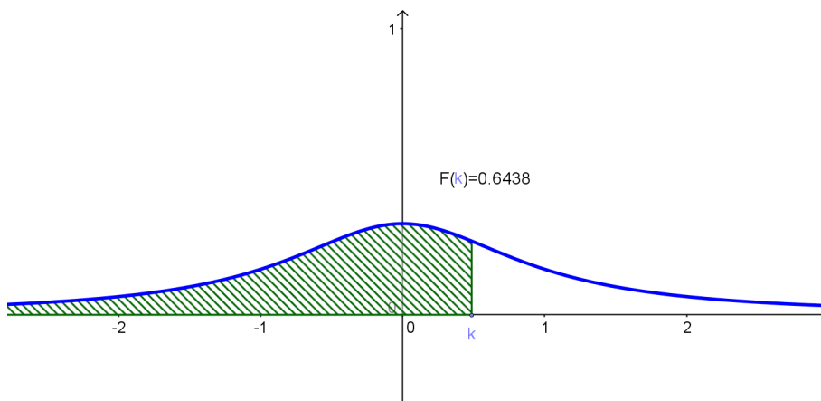
Figura 5.18: Cola izquierda de la distribución de X para el valor k \approx 0.486 . El área sombreada es F(k) = P(X \leq k)
