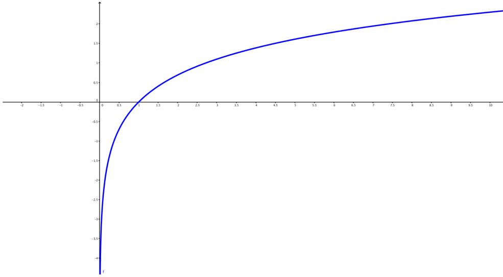
Figura 13.14: Transformación del intervalo (0, \infty) en el intervalo (-\infty, \infty) mediante el logaritmo.
