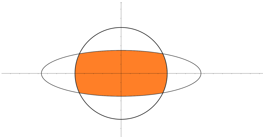
Figura 4.2: Un cálculo de probabilidad más complicado, para una variable aleatoria continua.
