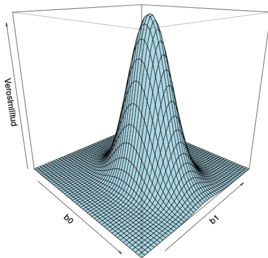
Figura 13.11: Función de máxima verosimilitud para los datos del Ejemplo 13.1.5.
