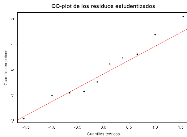
Figura 10.19: Gráficos para el análisis de los residuos en el Ejemplo 10.4.2
