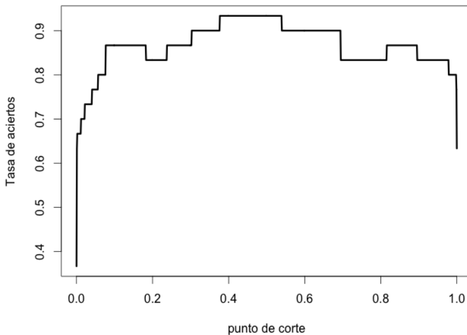
Figura 13.17: Tasa de aciertos en función del punto de corte c_p en el Ejemplo 13.7.9.
