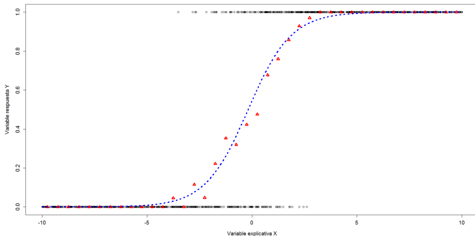
Figura 13.10: Construcción, por el método de mínimos cuadrados, de una curva logística para los datos del Ejemplo 13.1.5. ¡Esto no es regresión logística!
