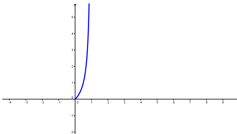
Figura 3.11: Relación entre probabilidad (en el eje horizontal) y posibilidades (odds, en el eje vertical).
