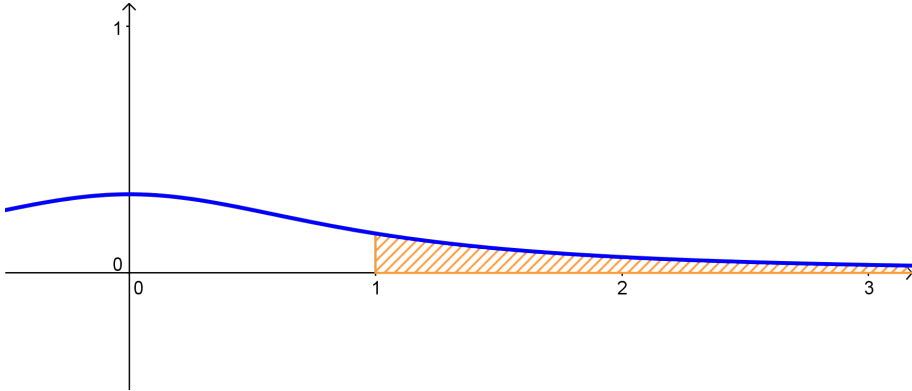
Figura 5.11: Cálculo de probabilidad para un intervalo no acotado.
