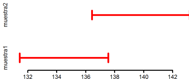
Figura 9.3: Intervalos de confianza para el segundo caso del Ejemplo 9.2.1
