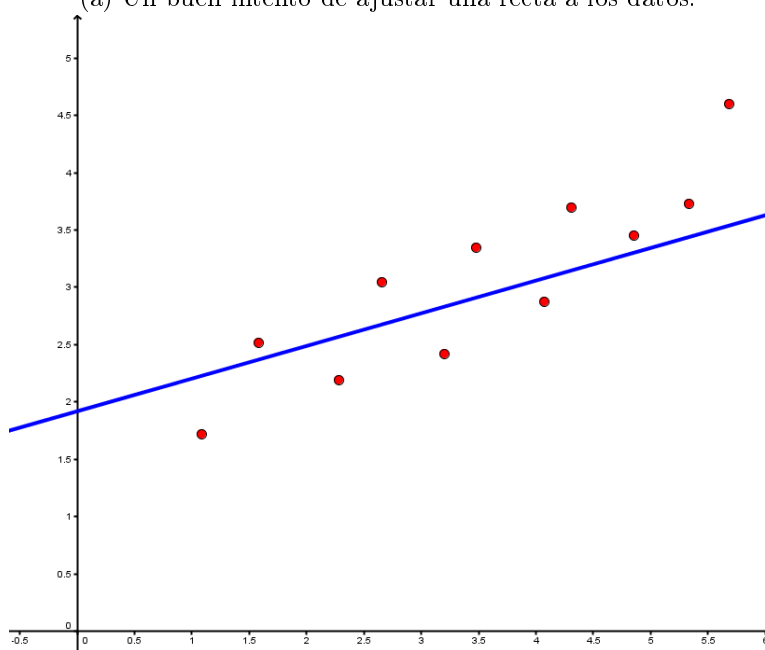
(b) Un intento bastante peor.
