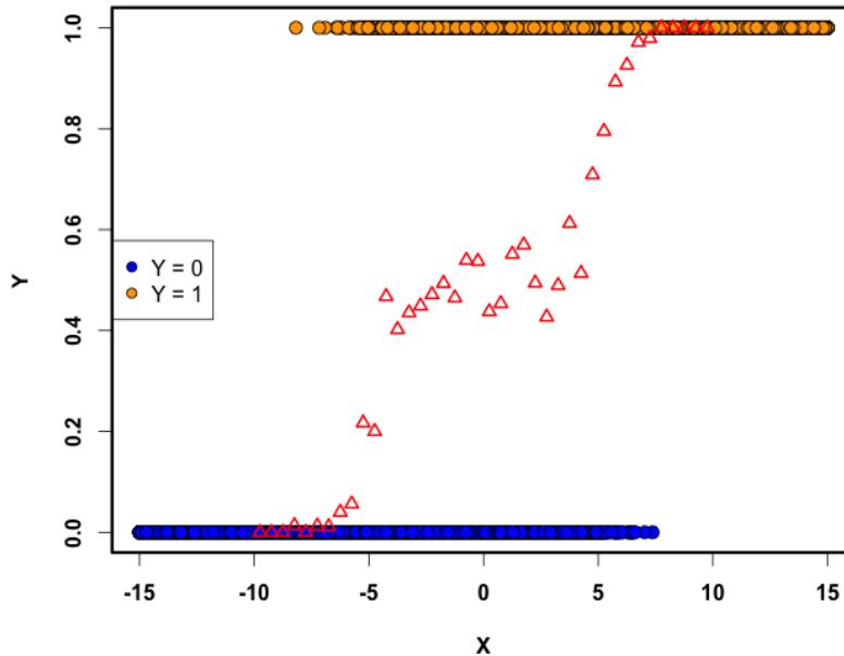
Figura 13.8: Los datos originales y los puntos (w_i, \hat{p}_i) del Ejemplo 13.1.6.
