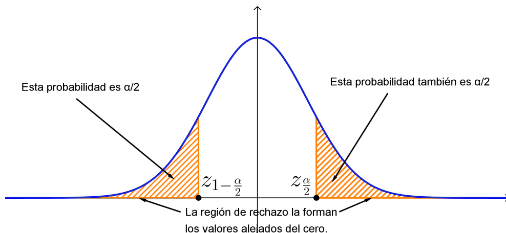
Figura 7.5: Región de rechazo para H_0 = \{\mu = \mu_0\} .
