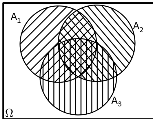
Figura 3.6: Diagrama para la intersección de tres sucesos.
