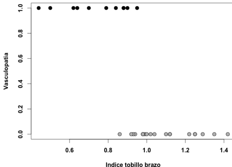
Figura 13.1: Datos muestrales, de la Tabla 13.1.
