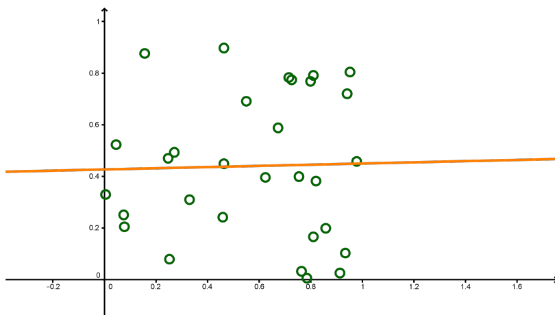
Figura 10.14: Otra razón por la que la recta de regresión puede ser de muy mala calidad.
