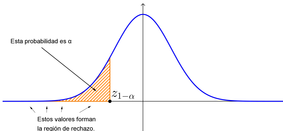
Figura 7.4: Región de rechazo para H_0 = \{\mu \geq \mu_0\} .
