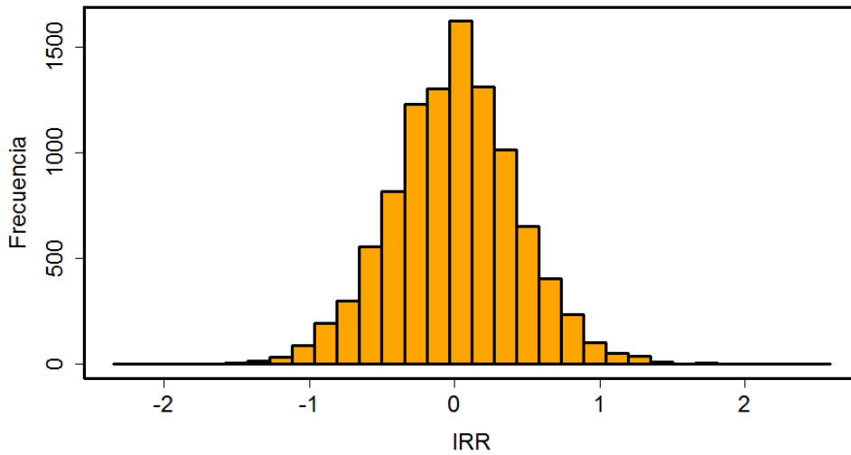
Figura 9.6: Simulación con 10000 muestras, de tamaño n = 50 , con p_1 = p_2 = 0.2 , en el Ejemplo 9.4.2. (a) Distribución muestral del riesgo relativo. (b) Distribución muestral del logaritmo del riesgo relativo.
