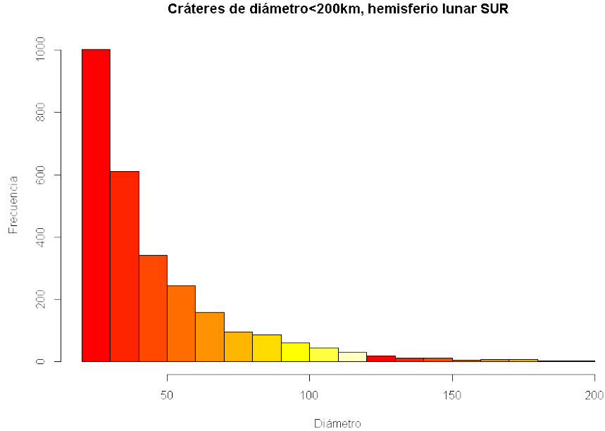
Figura 9.1: Distribución de diámetros (< 200 km), de cráteres del hemisferio sur lunar
