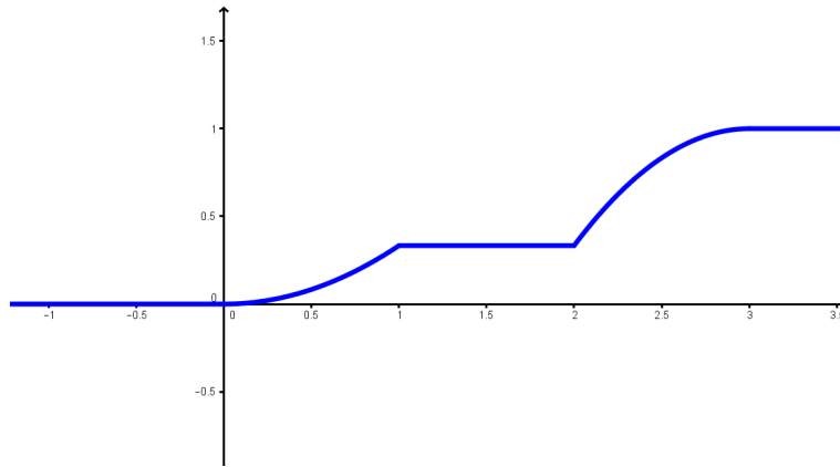
Figura 5.22: Gráfica de la función de distribución F(k) del Ejemplo 5.5.2.
