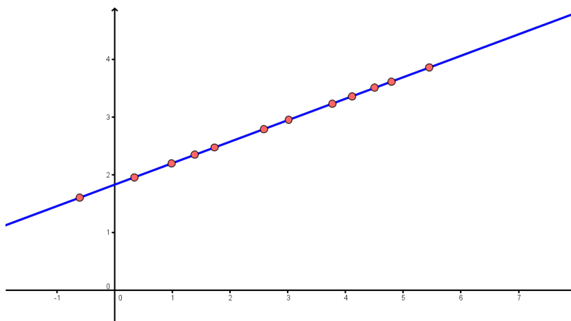
Figura 10.8: El único caso en el que EC = 0 es el de los puntos situados en una recta.
