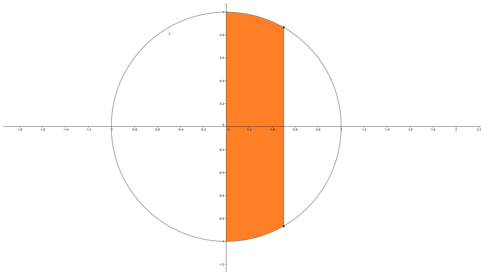
Figura 4.1: Cálculo de probabilidad en una variable aleatoria continua
