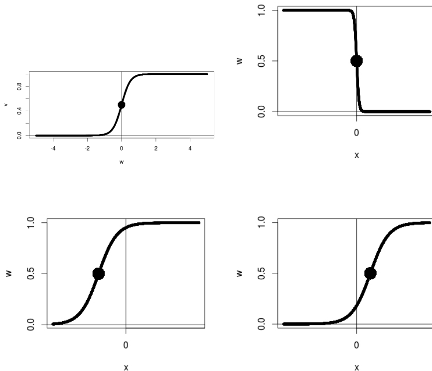
Figura 13.9: Curvas logísticas; arriba a la izquierda w = e^v/(1 + e^v) , arriba a la derecha w = e^{-8v}/(1 + e^{-8v}) , abajo a la izquierda w = e^{3+v}/(1 + e^{3+v}) , abajo a la derecha w = e^{-1.5+v}/(1 + e^{-1.5+v}) .
