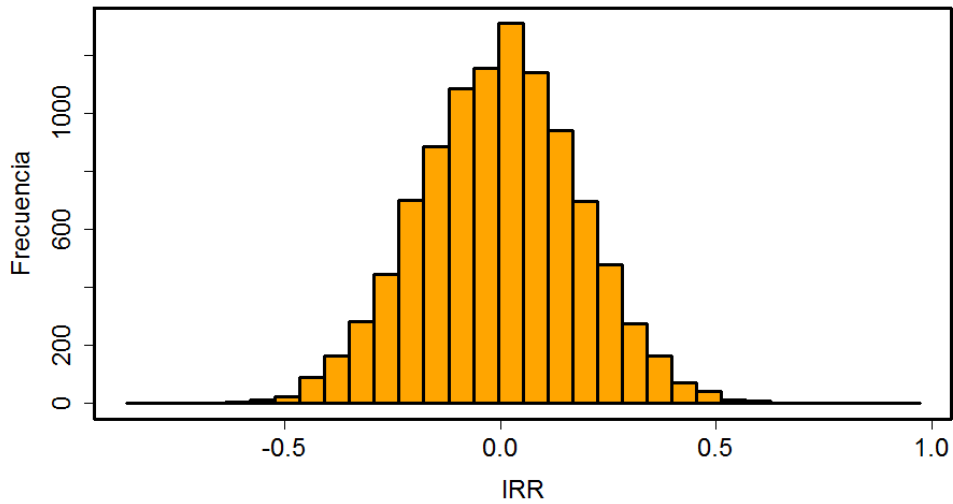
Figura 9.7: Simulación con 10000 muestras, de tamaño n = 250 , con p_1 = p_2 = 0.2 , en el Ejemplo 9.4.2. (a) Distribución muestral del riesgo relativo. (b) Distribución muestral del logaritmo del riesgo relativo.
