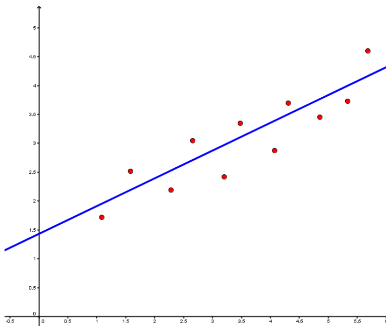
(a) Un buen intento de ajustar una recta a los datos.
