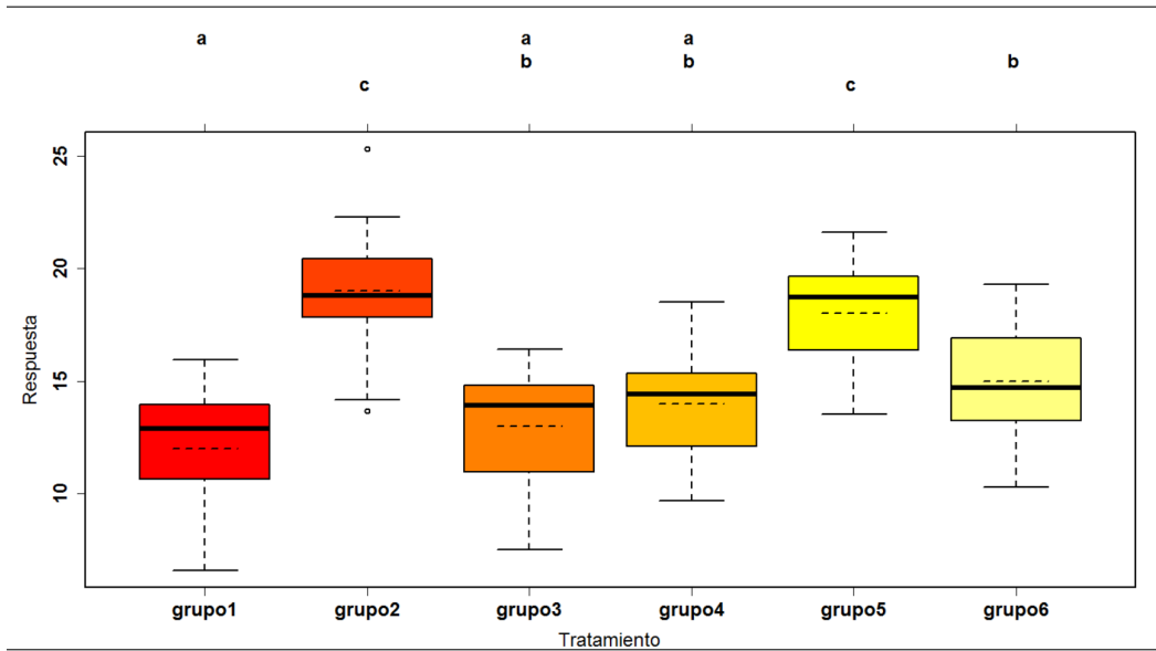
Figura 11.4: Comparaciones por parejas de las medias del Ejemplo 11.6.4. Los segmentos horizontales discontinuos indican la altura a la que se sitúan las medias de cada grupo.
