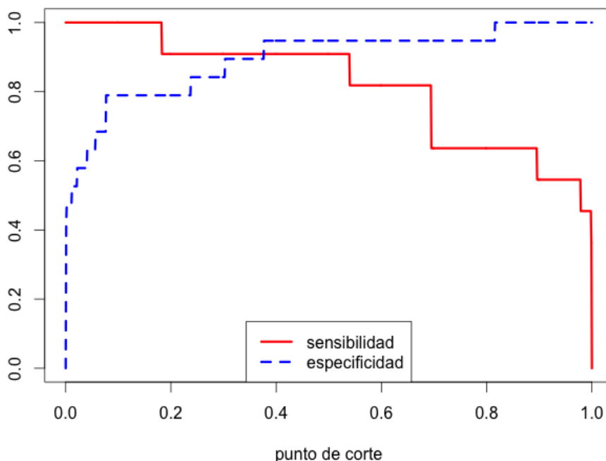
Figura 13.16: Sensibilidad y especificidad en función del punto de corte c_p en el Ejemplo 13.7.8.
