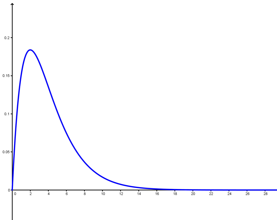
Figura 6.12: Función de densidad de la distribución \chi^2 con k = 4 grados de libertad.
