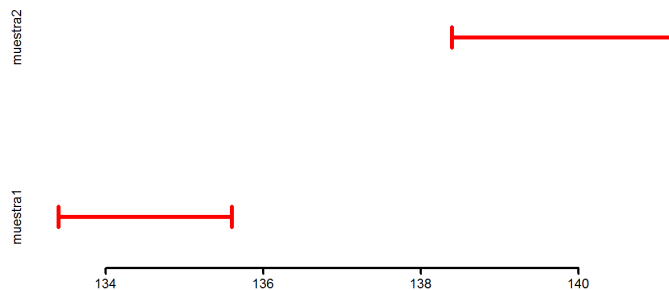
Figura 9.2: Intervalos de confianza para el primer caso del Ejemplo 9.2.1
