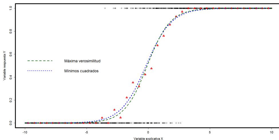
Figura 13.12: Las curvas logísticas obtenidas por el método de mínimos cuadrados (puntos, color azul) y por el método de máxima verosimilitud (trazos verdes), para los datos del Ejemplo 13.1.5.
