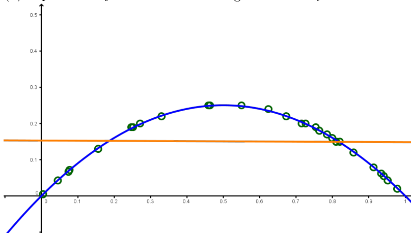
Figura 10.13: Un ejemplo de recta de regresión de muy mala calidad.
