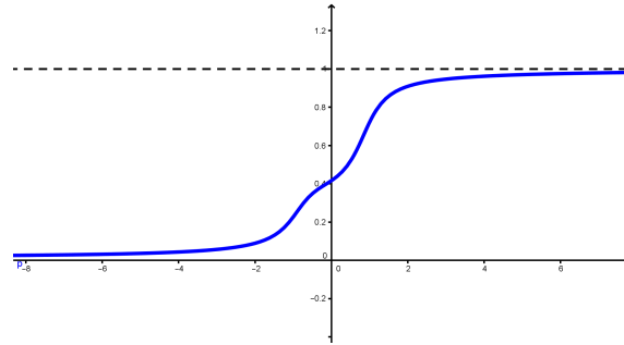
Figura 5.20: Una “típica” función de distribución de una variable aleatoria continua.
