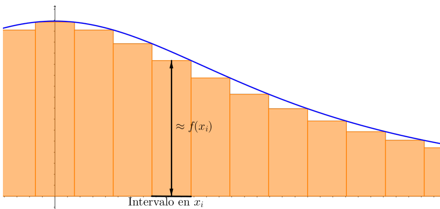
Figura 5.17: Detalles de la discretización de una variable aleatoria continua
