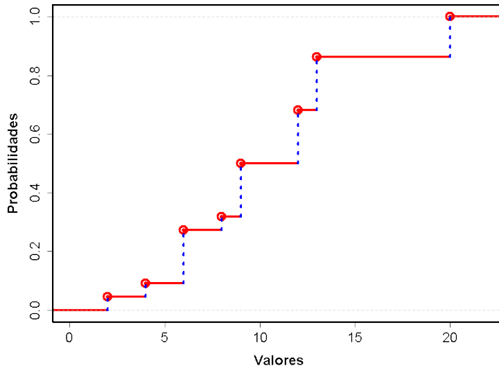
Figura 4.3: Una “típica” función de distribución de una variable aleatoria discreta
