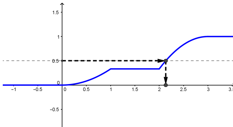
Figura 5.23: Buscando la mediana de la variable X del Ejemplo 5.5.2.
