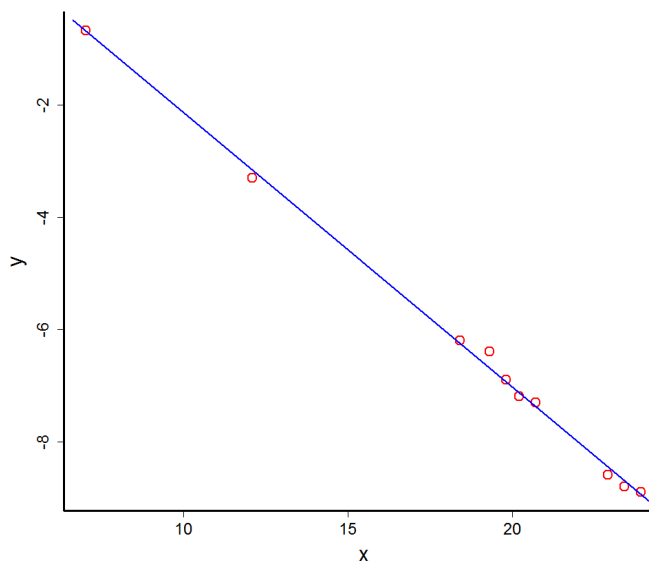
Figura 10.9: Puntos y recta de regresión del Ejemplo 10.2.1.
