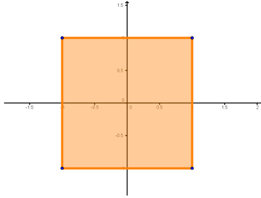
Figura 5.28: Suceso A en el Ejemplo 5.7.1.
