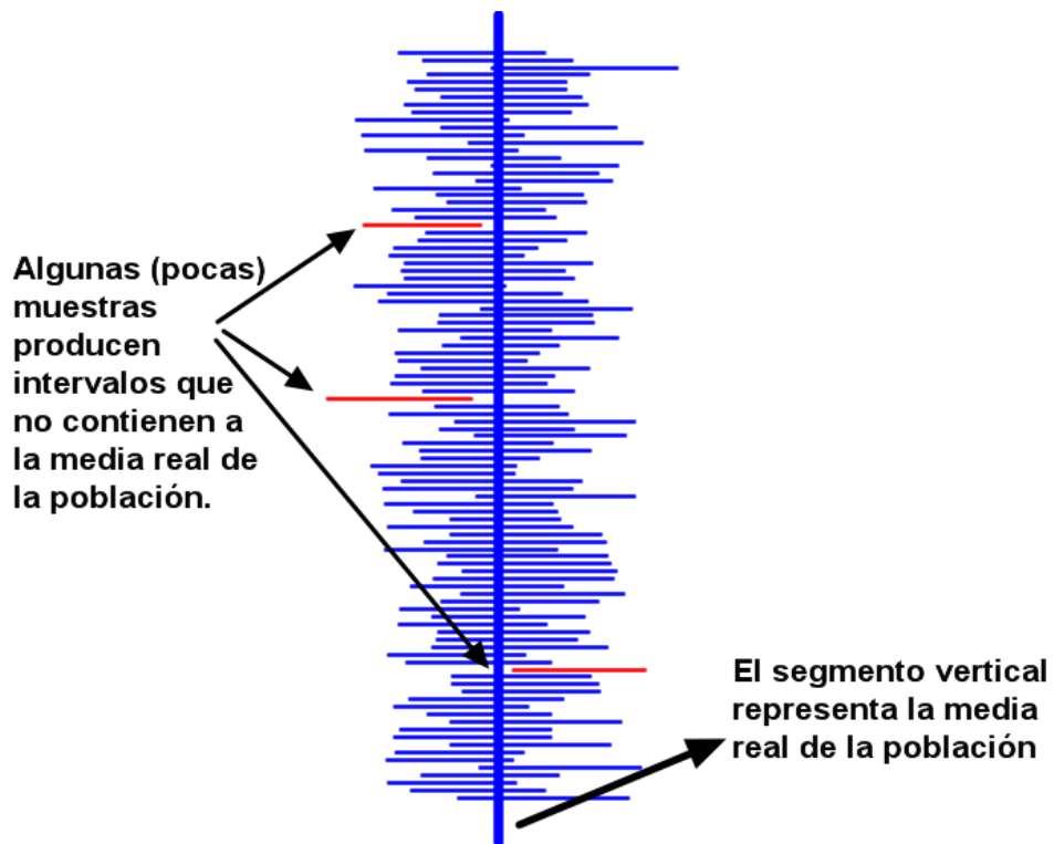
Figura 6.9: Interpretación probabilística de los intervalos de confianza.
