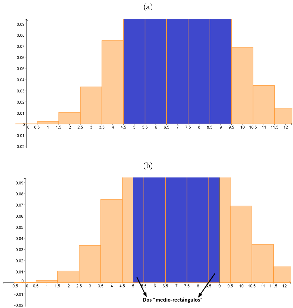
Figura 5.25: (a) Detalle de la aproximación binomial normal (b) Justificación de la corrección de continuidad
