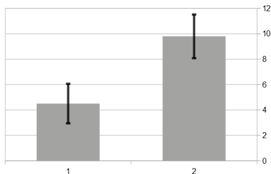
Figura 9.4: Gráfico con barras de error estándar de la media. ¡SE DESACONSEJA EL USO DE ESTE TIPO DE GRÁFICOS!
