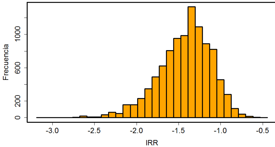
Figura 9.8: Simulación con 10000 muestras, de tamaño n = 50 , con p_1 = 0.2 y p_2 = 0.8 , en el Ejemplo 9.4.2. (a) Distribución muestral del riesgo relativo. (b) Distribución muestral del logaritmo del riesgo relativo.
