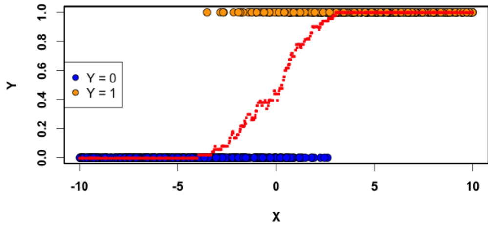
Figura 13.15: Estimaciones de probabilidad por el método de clasificación knn en el Ejemplo 13.7.6. En la parte (a) se ha usado k = 5 , mientras que en la parte (b) usamos k = 100 .
