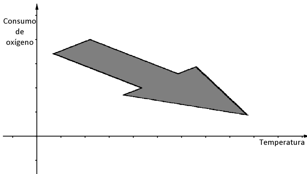
Figura 10.2: Nuestra intuición sobre la relación entre las dos variables en el problema de los herrerillos.
