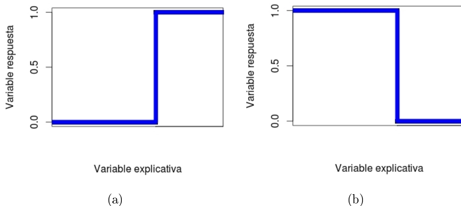
Figura 13.2: Gráficas de las funciones escalón: (a) directa y (b) inversa.
