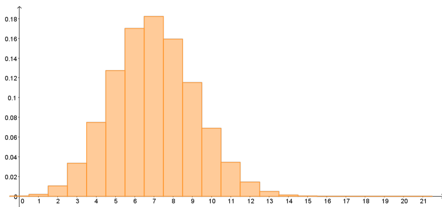
Figura 5.5: Distribución binomial n = 21 , p = \frac{1}{3} .
