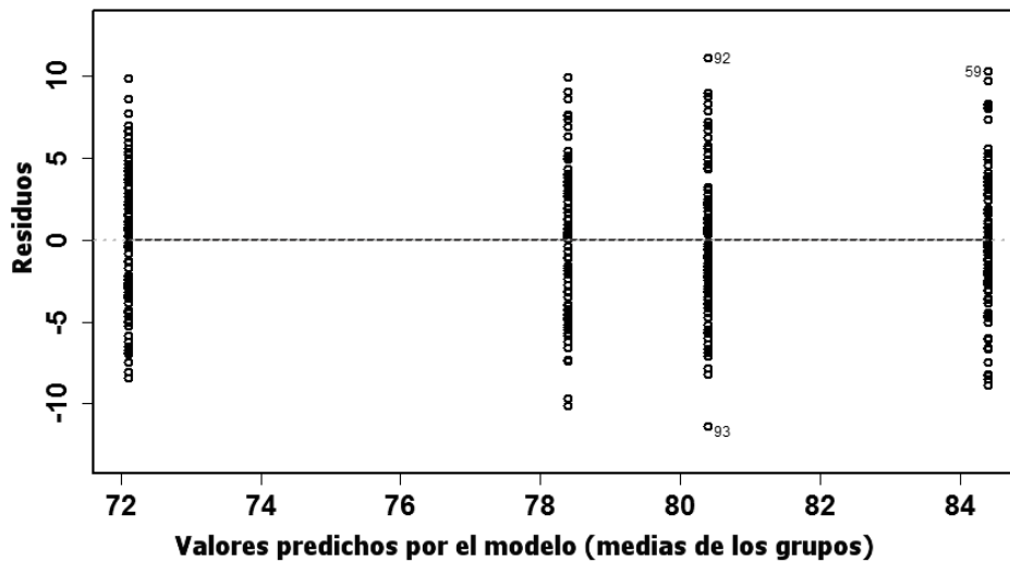
Figura 11.2, continuación. (c) QQ-plots por grupos (d) Residuos frente a valores predichos por el modelo.
