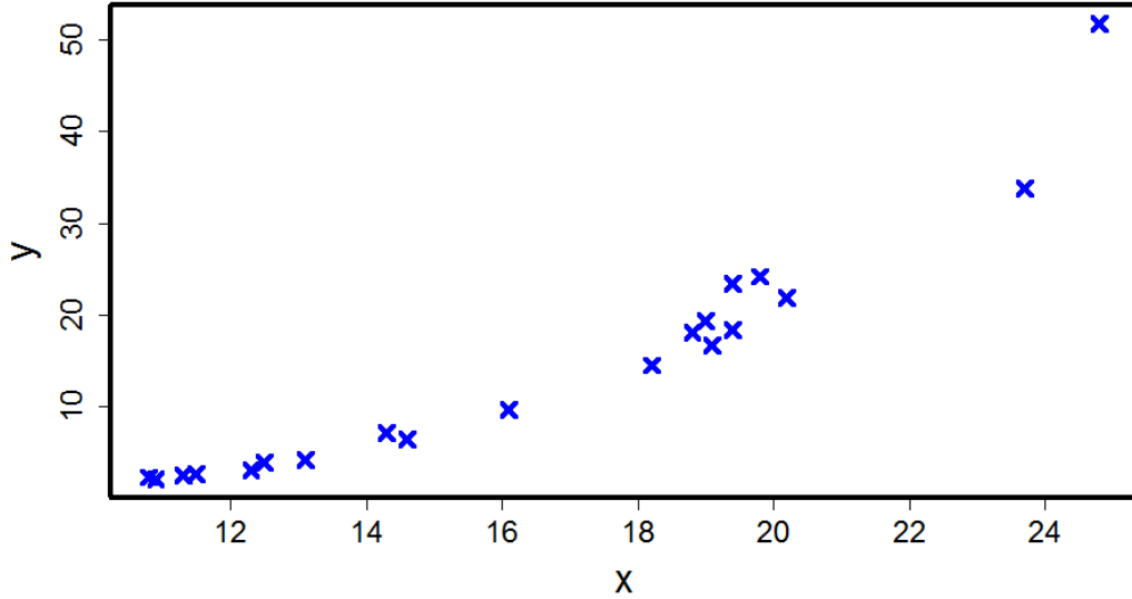
captionDiagrama de dispersión del Ejemplo 10.5.1
