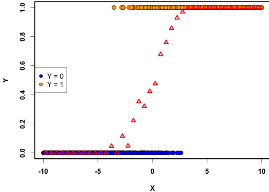
Figura 13.7: Predicción de probabilidades por clases para el Ejemplo 13.1.5.
