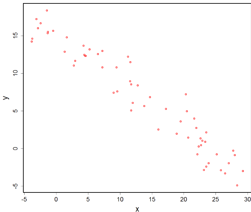
Figura 10.3: Diagrama de dispersión (con datos simulados) para el experimento del Herre-rillo incubando. El eje x representa la temperatura y el eje y el consumo de oxígeno, en las unidades adecuadas.
