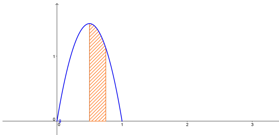
Figura 5.15: El área sombreada es P\left(\frac{1}{2} < X < \frac{3}{4}\right)
