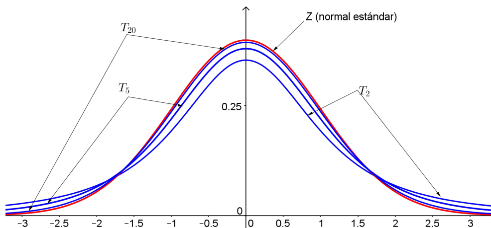
Figura 6.10: La normal estándar Z , comparada con distribuciones T_k de Student, para distintos valores de k .
