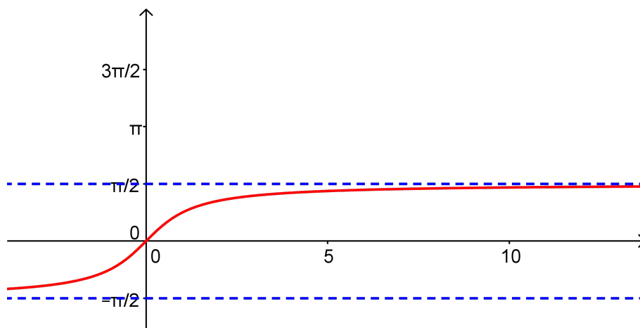
Figura 5.10: Gráfica de la función \arctan(x) para el Ejemplo 5.4.3.
