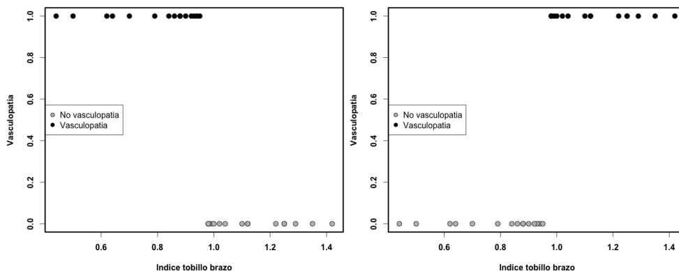
Figura 13.3: Situación idealizada del Ejemplo 13.1.4.
