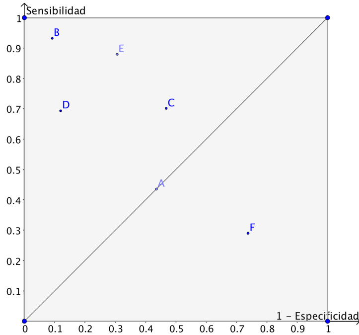
Figura 13.18: El espacio de coordenadas (1 - especificidad, sensibilidad) que se usa para comparar clasificadores.
