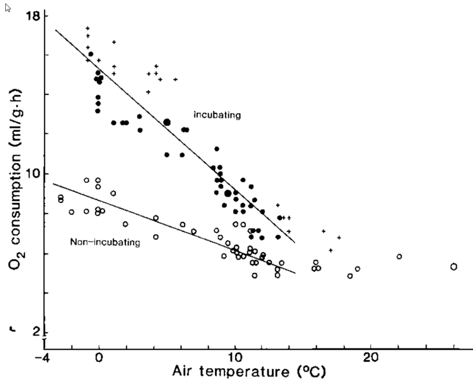
Figura 10.5: Reproducción de la Figura 5 del artículo [HR85] de S. Haftorn y R. E. Reinertsen, "The effect of temperature and clutch size on the energetic cost of incubation in a free-living blue tit ( parus caeruleus )", The Auk , pp. 470–478, 1985.. La figura aparece en la pág. 473. El pie de la figura dice: Relación entre la tasa de consumo de oxígeno de una hembra de Herrerillo Común cuando está en pie sobre los huevos, sin incubarlos (círculos abiertos), y cuando está incubando 13 huevos (círculos sólidos) [...]. Recta de regresión superior ( n = 71 ): y = 15.35 - 0.62x . Recta de regresión inferior( n = 41 ): y = 8.45 - 0.22x . Datos de 1983.
