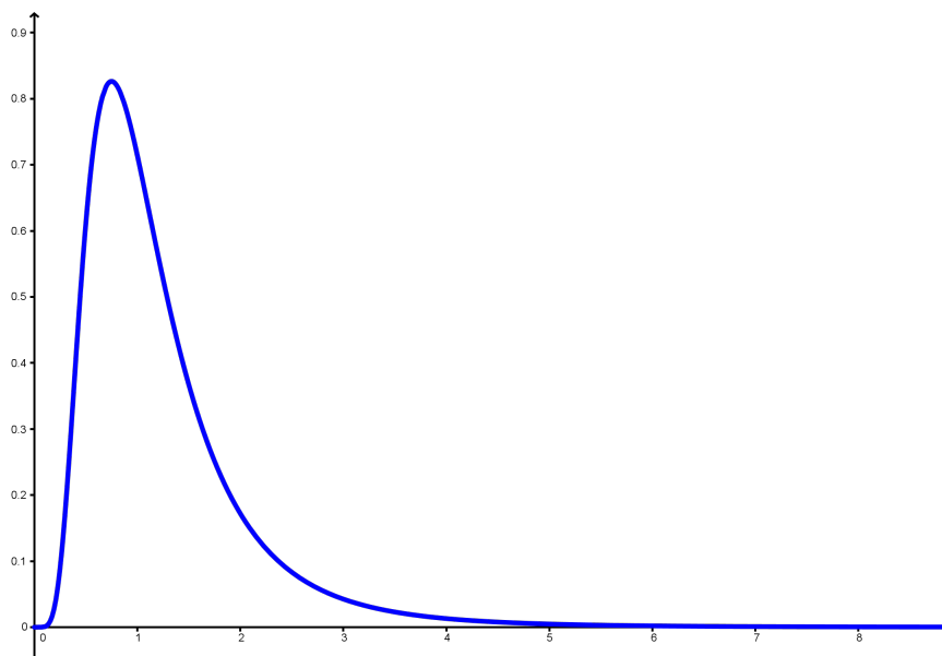
Figura 9.5: Función de densidad de la distribución F_{20,10}
