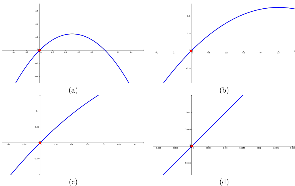
Figura 10.10: La recta como aproximación local, en este caso a la parábola y = x - x^2 . Al aumentar el zoom en el origen, la parábola se parece cada vez más a su recta tangente en el origen.
