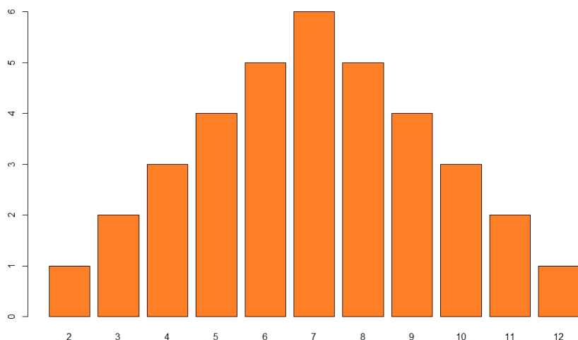
Figura 6.2: Distribución de la variable X , suma al lanzar dos dados.
