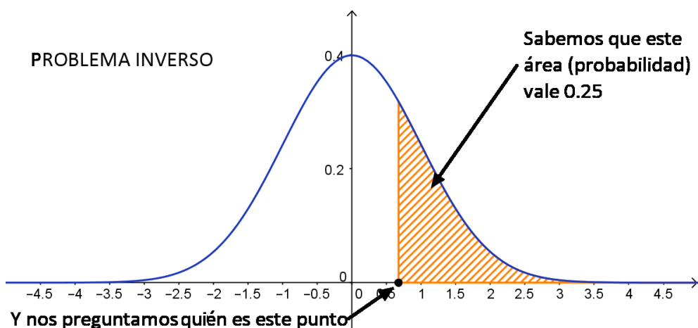
Figura 6.6: Un problema inverso de probabilidad en Z .
