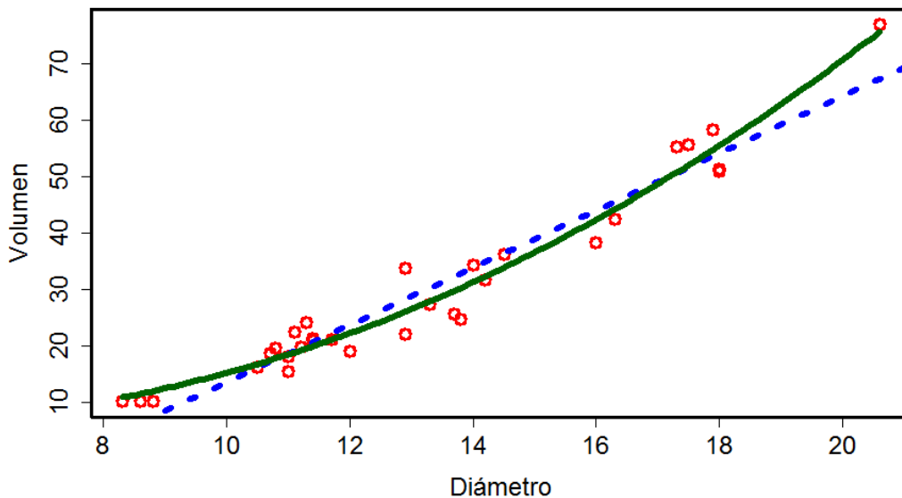
Figura 10.28: Polinomio cuadrático de regresión (línea continua) y recta de regresión (a trazos), para los datos del Ejemplo 10.5.3.
