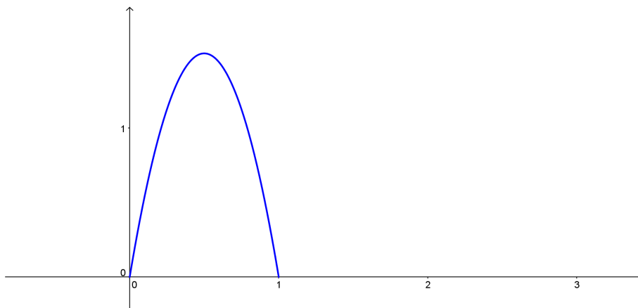
Figura 5.14: Una función de densidad que sólo es \neq 0 en (0, 1) .
