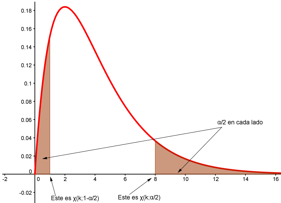
Figura 6.15: Valores críticos en la construcción de un intervalo de confianza para \sigma^2 , usando \chi_k^2 .
