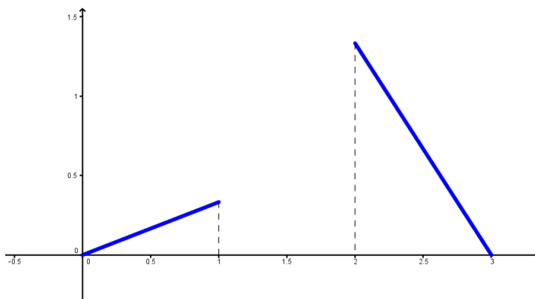
Figura 5.21: Gráfica de la función de densidad del Ejemplo 5.5.2.
