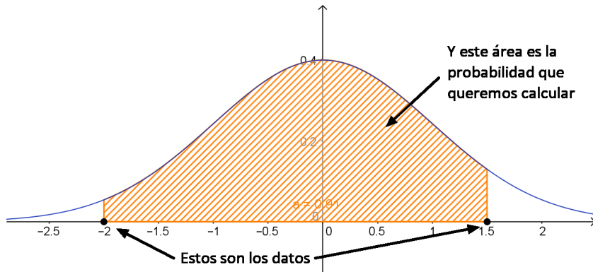
Figura 6.4: Un problema directo de probabilidad en Z .
