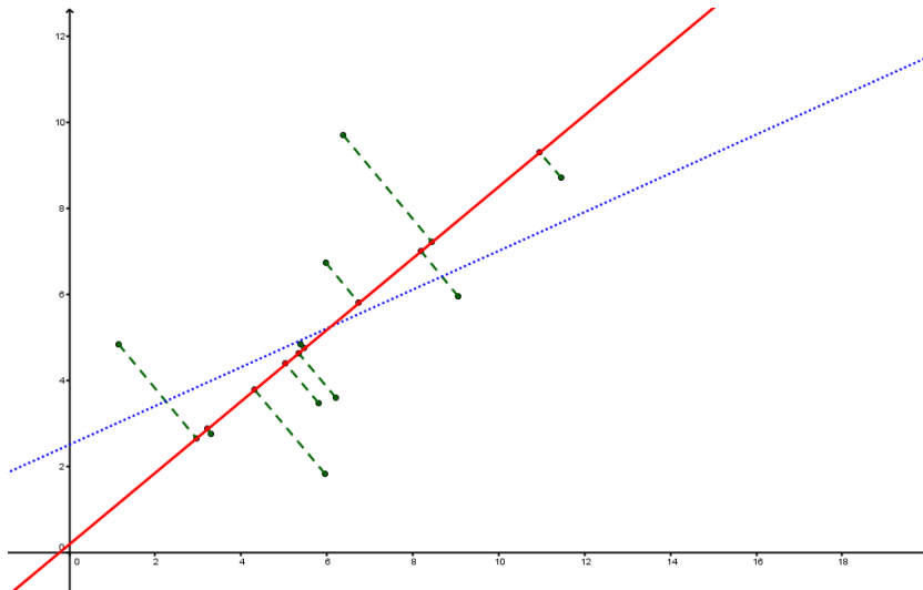
Figura 10.12: Recta de regresión ortogonal (major axis, en trazo continuo) y recta de regresión por mínimos cuadrados (trazo a puntos), para el mismo conjunto de puntos.
