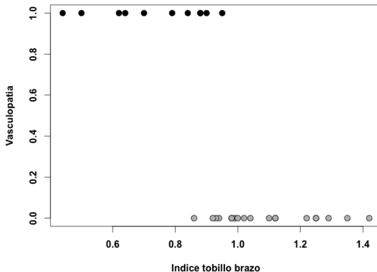
Figura 13.4: Datos muestrales, de la Tabla 13.1.
