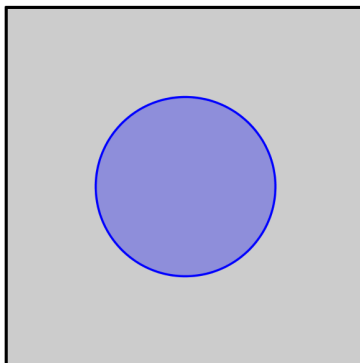
Figura 3.2: Círculo de radio 1 centrado en un cuadrado de lado 4.
