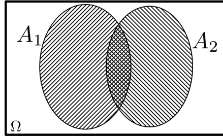
Figura 3.4: Diagrama para la intersección de dos sucesos
