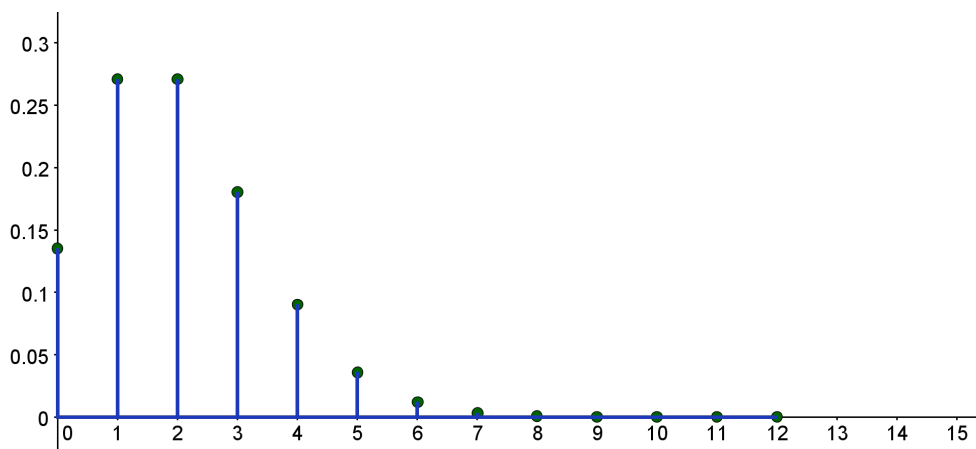
Figura 8.2: Valores de probabilidad de la distribución de Poisson con \lambda = 2 . Los valores correspondientes a k > 12 son muy pequeños, y no se muestran.
