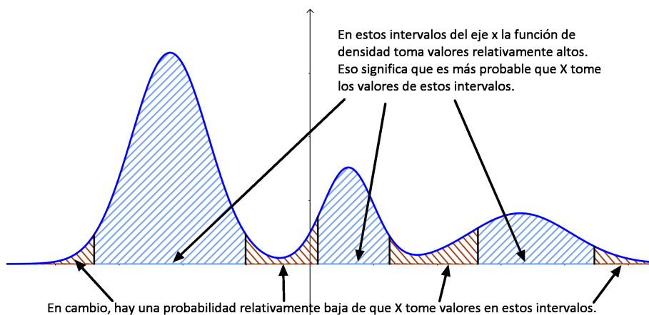
Figura 5.13: La altura de la función de densidad indica los valores de X con más probabilidad.
