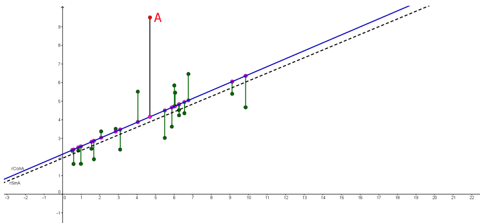
(b) El punto A no es influyente, con residuo atípico, pero palanca muy pequeña.
