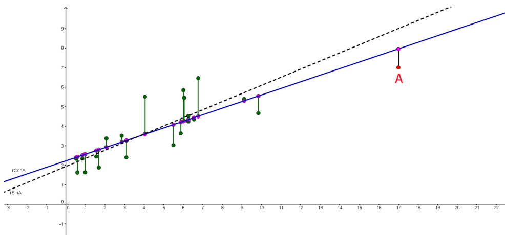
(a) El punto A es influyente, con palanca grande y residuo moderado.
