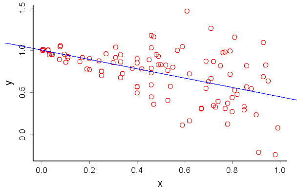
Figura 10.21: El diagrama inicial de dispersión de x frente a y correspondiente a la parte (b) de la Figura 10.20.
