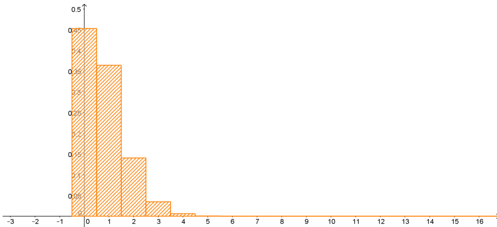
Figura 5.26: Distribución binomial con p pequeño; se representa n = 26, p = 0.03 .
