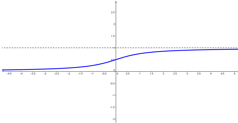
Figura 5.19: Función de distribución F(k) del ejemplo 5.5.1
