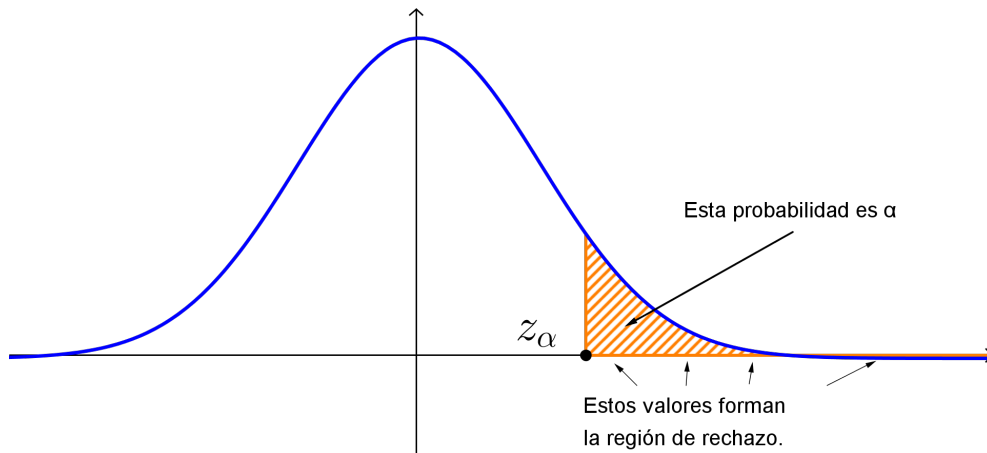
Figura 7.3: Región de rechazo para H_0 = \{\mu \leq \mu_0\} .
