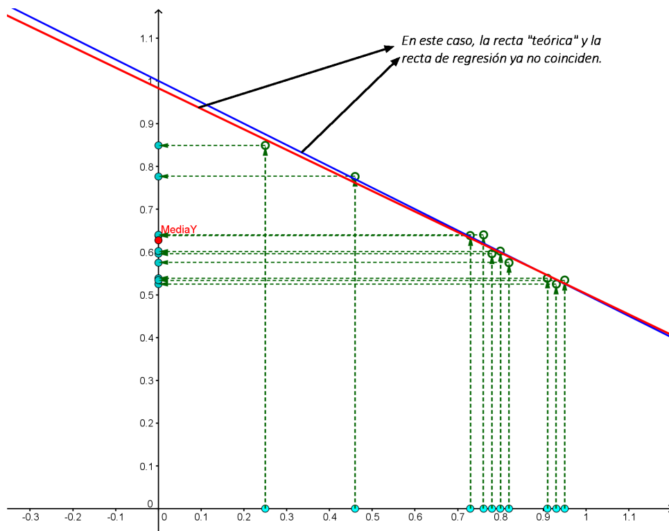
Figura 10.16: Anova en la regresión. Caso “ruidoso”: ahora la dispersión de y no se explica completamente por el efecto de la recta, y es necesario tener en cuenta el componente aleatorio que interviene en la generación de los valores y_i .
