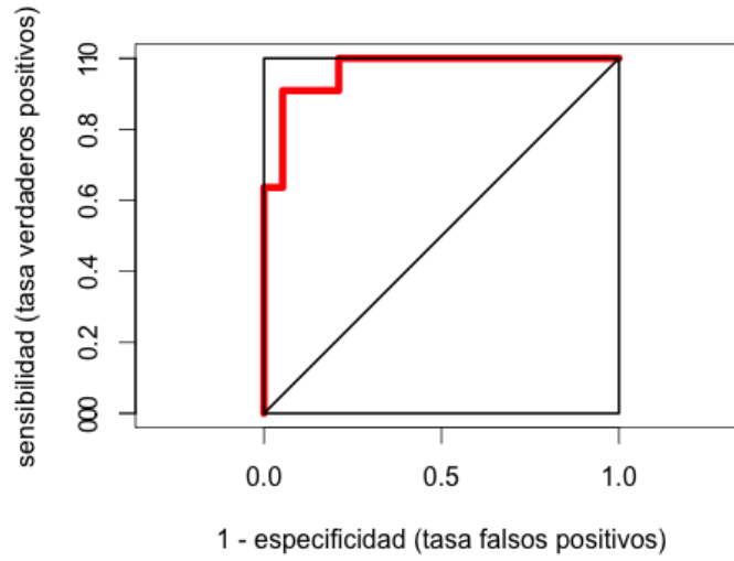
Figura 13.19: La curva ROC del Ejemplo 13.7.12.
