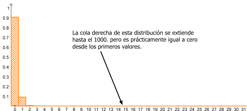
Figura 5.2: Distribución Binomial: B\left(1000, \frac{1}{10000}\right) .
