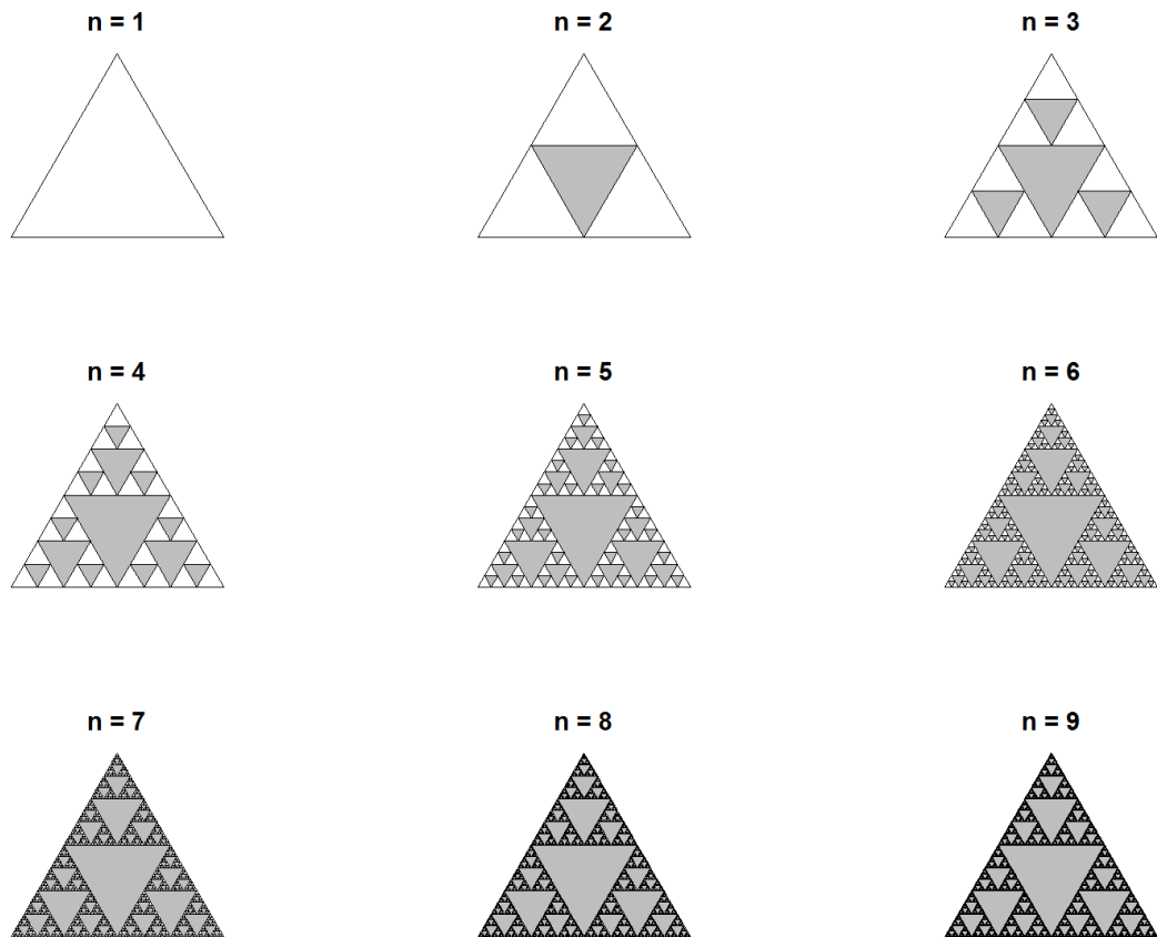
Figura 3.3: Las primeras etapas en la construcción del triángulo de Sierpinski
