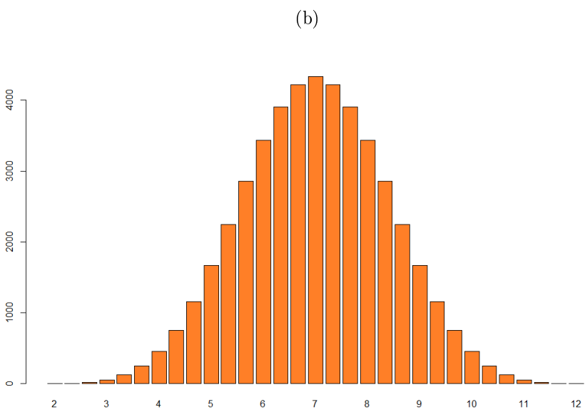
Figura 6.3: (a) Distribución de la variable original X y (b) de su media muestral \bar{X} .
