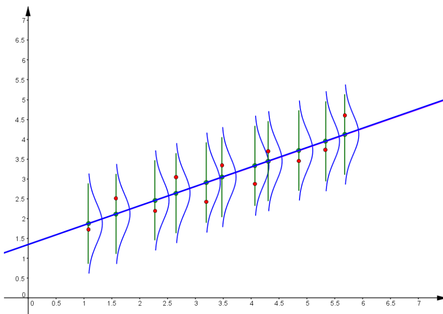
Figura 10.18: Ilustración del modelo de regresión lineal simple.
