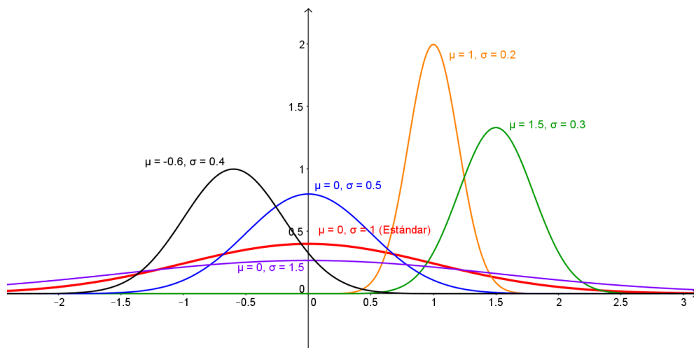
Figura 5.24: Curvas normales, para distintos valores de \mu y \sigma
