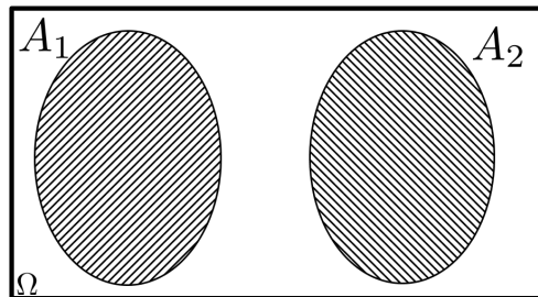
Figura 3.5: Dos sucesos incompatibles o disjuntos.
