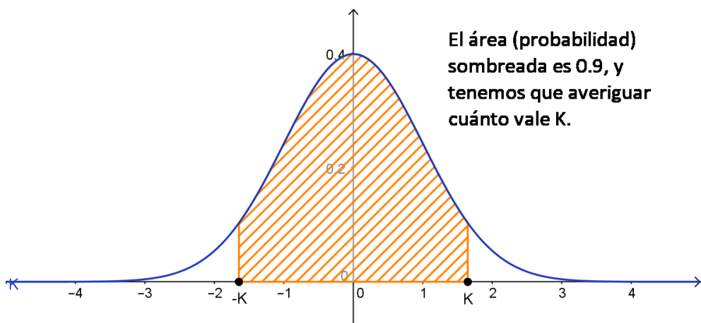
Figura 6.7: El paso clave en la construcción de un intervalo de confianza al 90 %.
