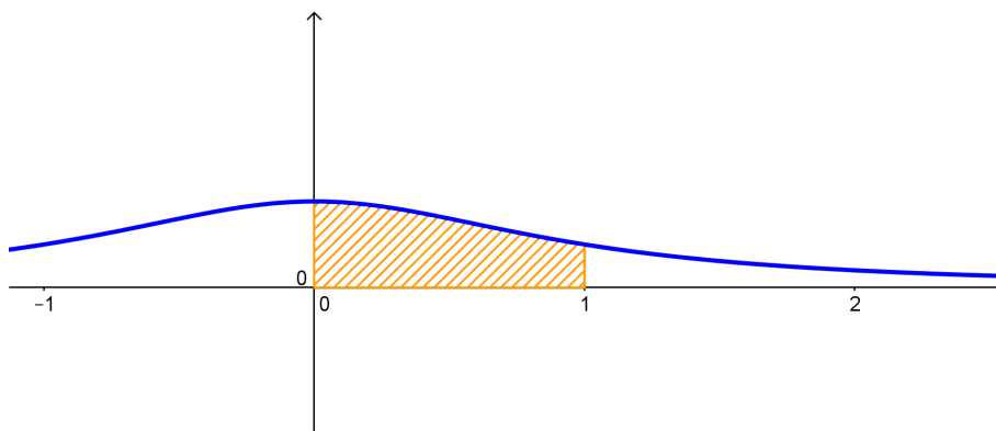
Figura 5.9: La probabilidad P(0 \leq X \leq 1) se calcula integrando f(x) entre 0 y 1.
