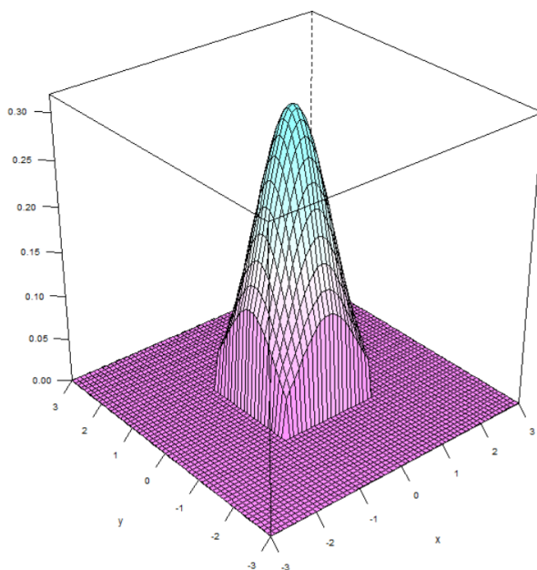
Figura 5.29: La probabilidad del suceso A del Ejemplo 5.7.1 es el volumen bajo la gráfica de f , y sobre el cuadrado que define A .
