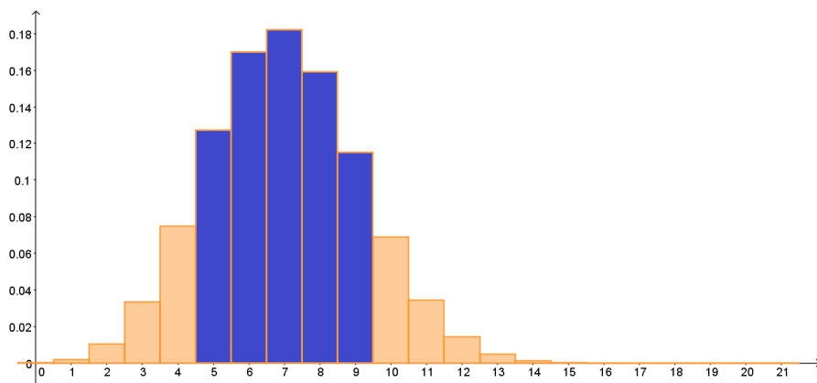
Figura 5.6: Probabilidad P(5 \leq X \leq 9) en la Distribución Binomial B(21, \frac{1}{3}) .
