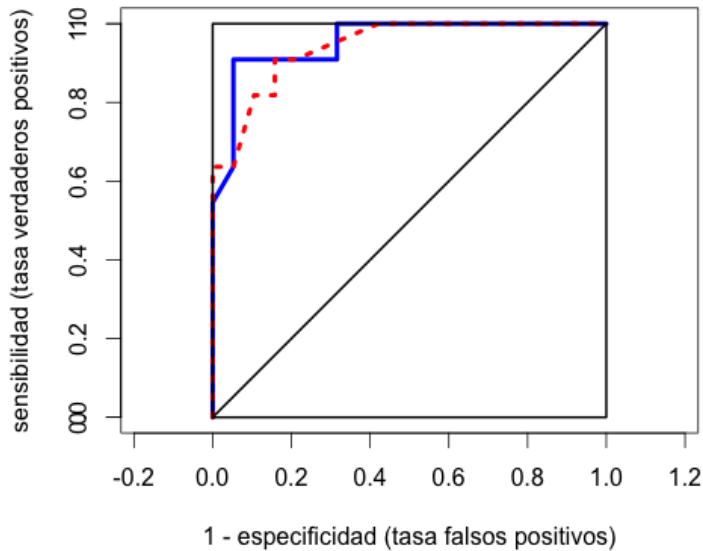
Figura 13.20: Curvas ROC para comparar dos clasificadores en el Ejemplo 13.7.12.
