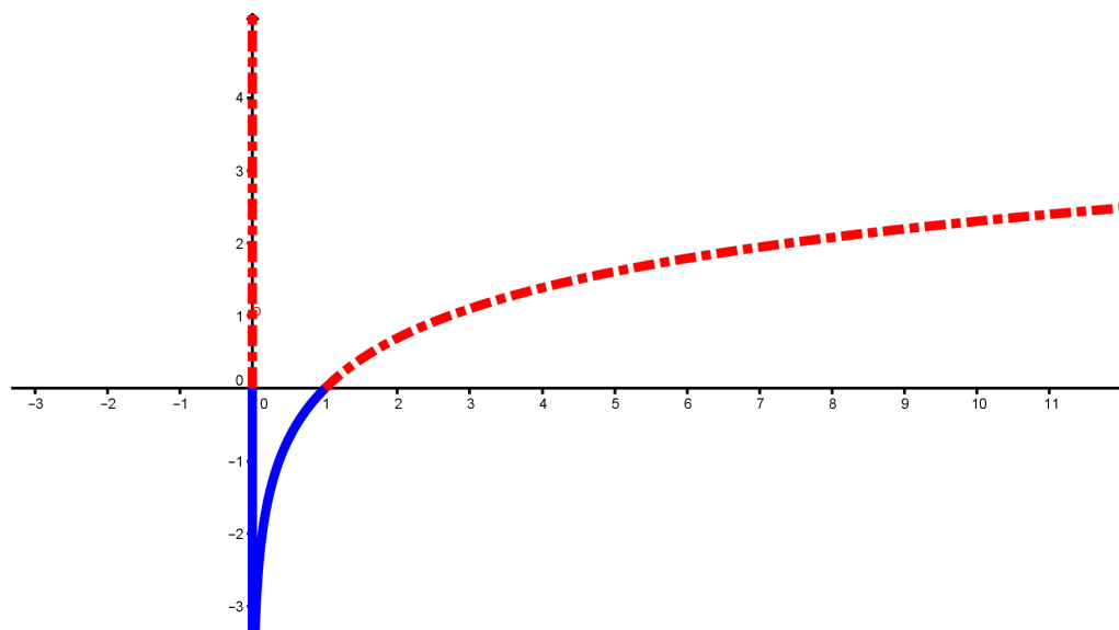
Figura 9.9: El logaritmo, y su efecto como transformación de datos.
