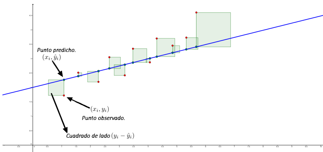
Figura 10.7: Interpretación geométrica del error cuadrático. La recta es una recta cualquiera.
