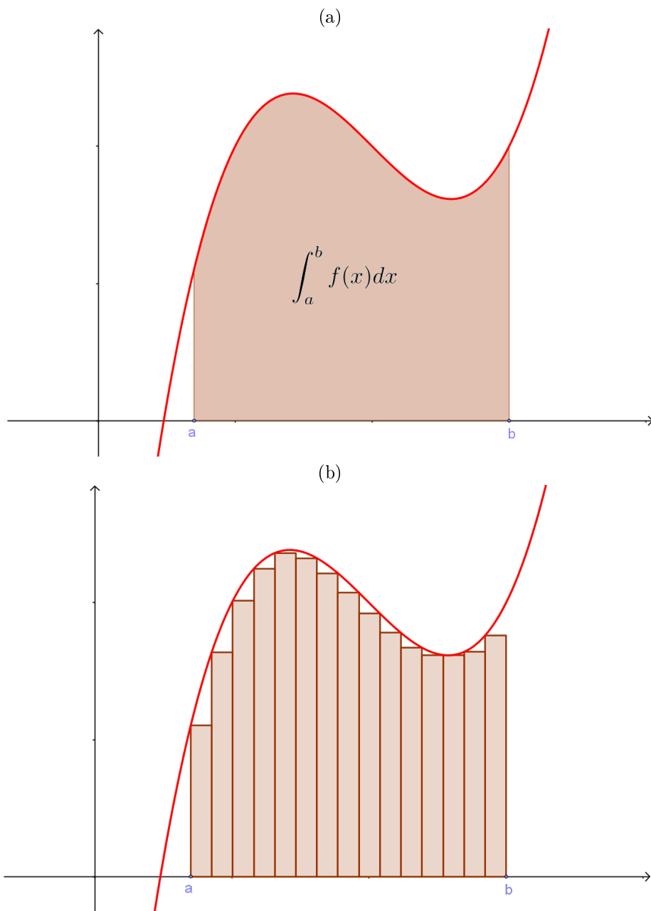
Figura 5.7: Newton mostró como relacionar (a) el área bajo una curva (una integral) con (b) una suma de áreas de rectángulos cada vez más numerosos y estrechos.
