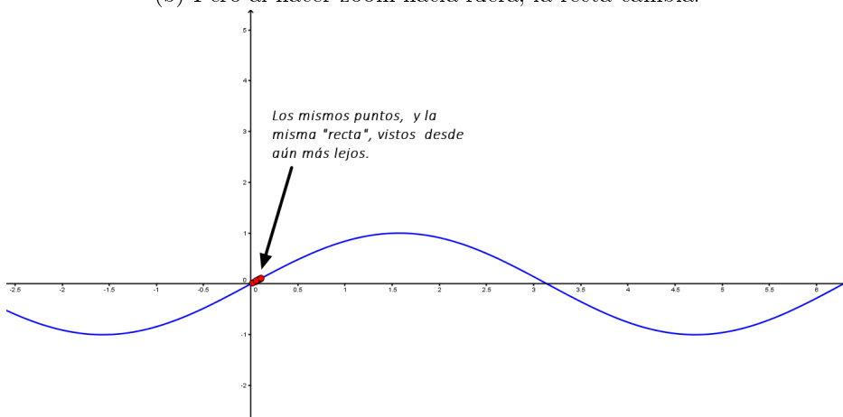
Figura 10.11: La recta como aproximación local a una función.
