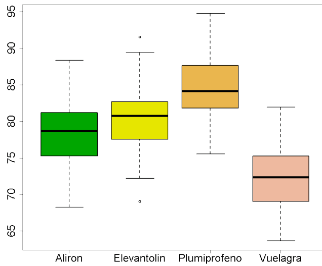
Figura 11.2: (a) Histogramas y (b) diagramas de cajas paralelos para la condición de normalidad.
