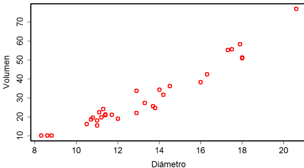
Figura 10.27: Diagrama de dispersión de los datos del Ejemplo 10.5.3.
