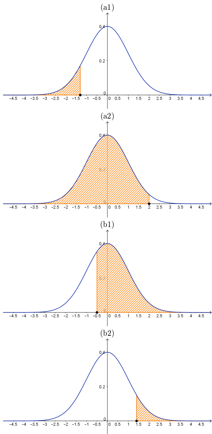
Figura 6.5: Problemas (directos) de probabilidad sobre colas de Z . Los dos primeros son colas izquierdas: (a1) P(Z < -1.3) , (a2) P(Z < 2) . Los dos últimos, colas derechas: (b1) P(Z > -0.5) , (b2) P(Z > 1.4) . En todos los casos, queremos calcular el área sombreada.
